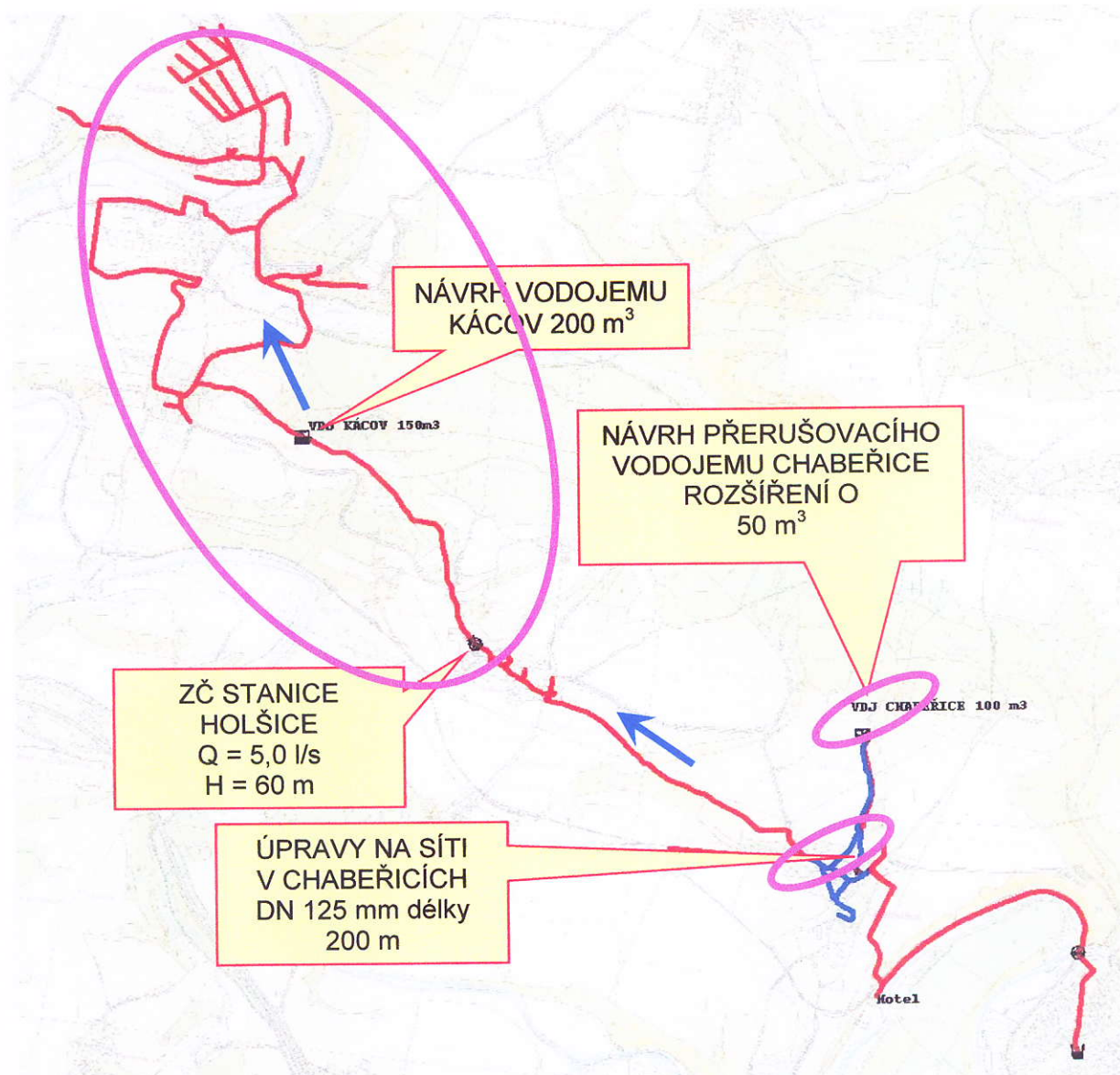
Situace vodovod Kácov (ohraňeno fialově) a vodovod Chabeřice
